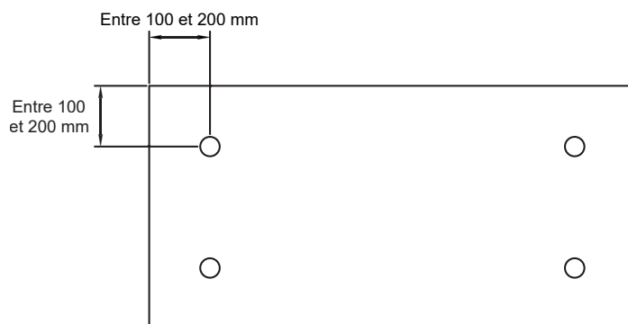
Figure 2 - Schéma de principe de la mise en œuvre des fixations des panneaux de dimensions maximales 1 200 mm x 1 000 mm
