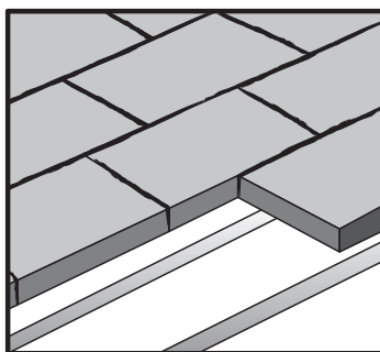
Figure 5 - Sens de pose des panneaux en verre cellulaire sur TAN
